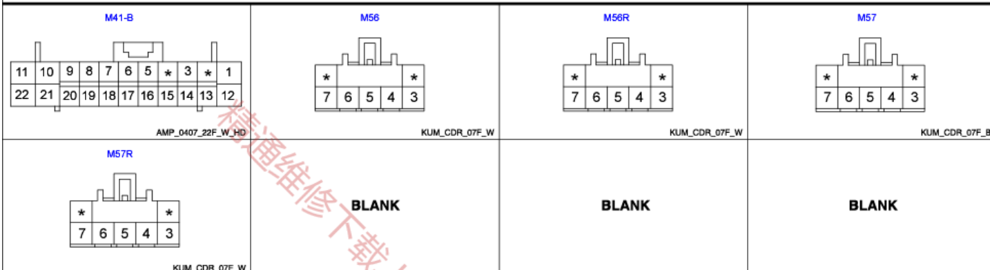
前鼓风机 &amp; 空调控制系统（自动）（7）
